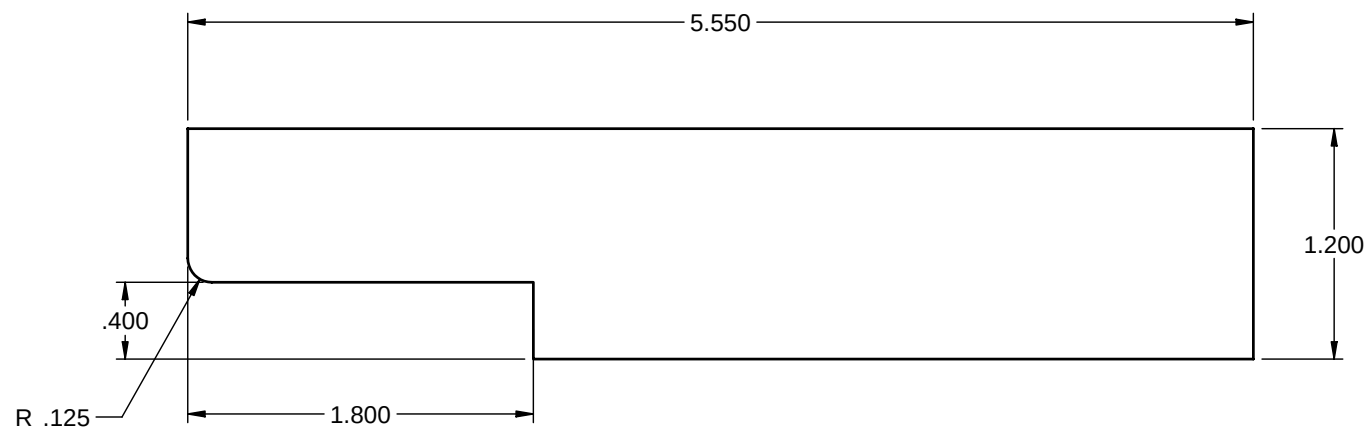
LEFT SIDE
