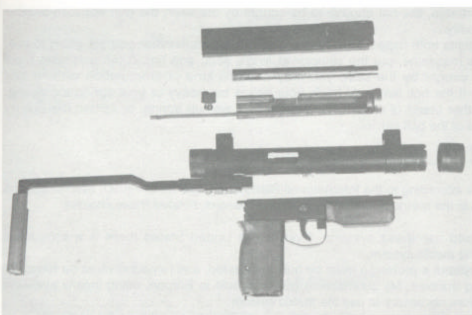
Field-stripped Métral.
