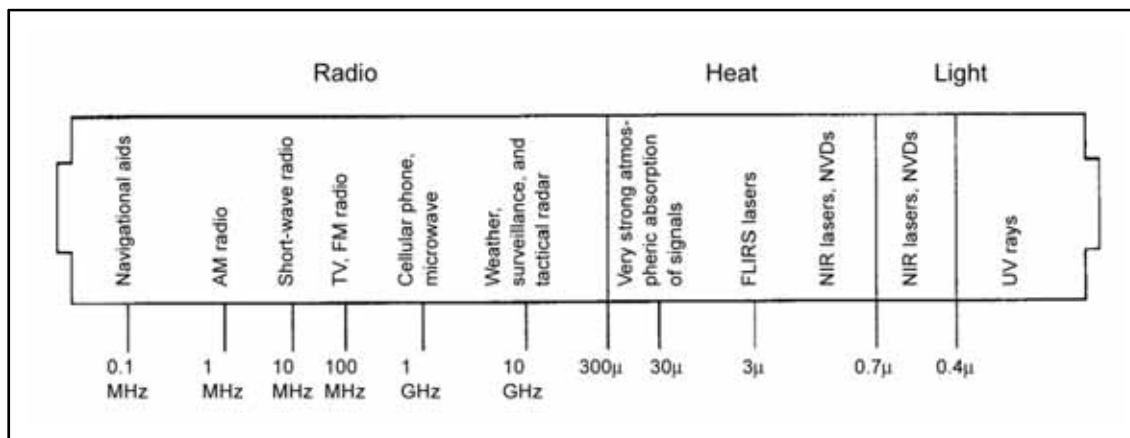
Figure 2-1. EM spectrum
