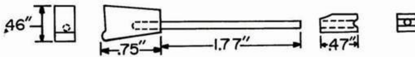
Fig. 5-13 MAINSPRING STRUT
