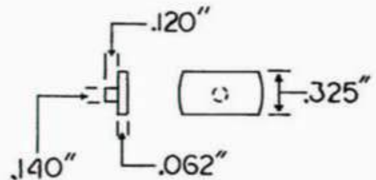
Fig. 3-15 PIVOTAL BAR
