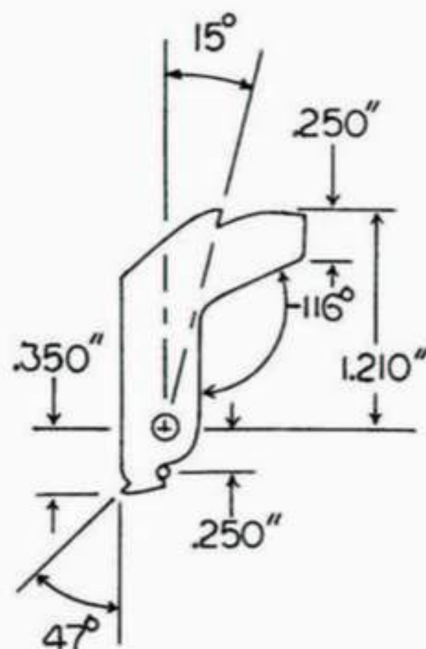
Fig. 3-21 HAMMER
