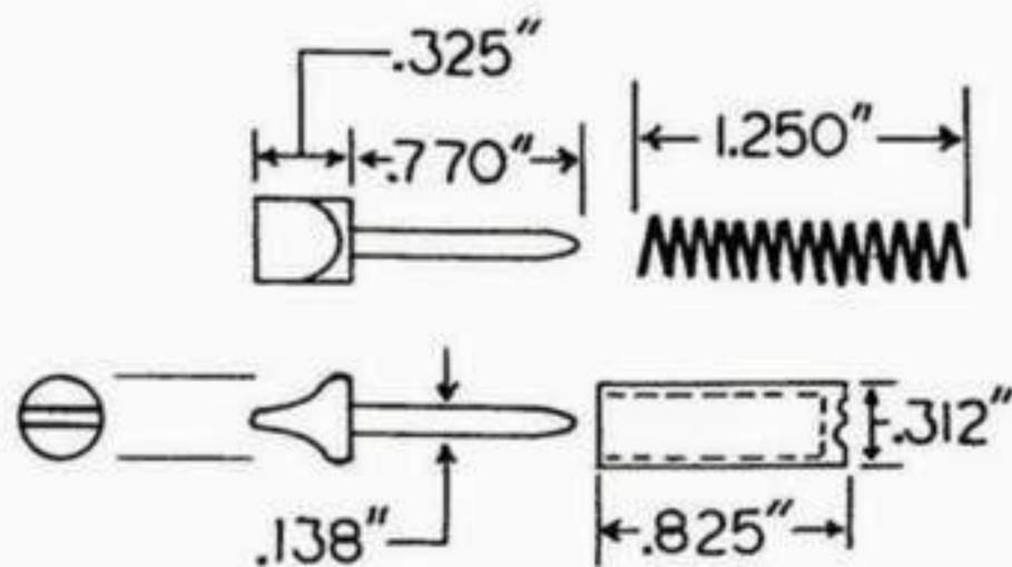
Fig. 3-22 MAINSPRING PLUNGER
