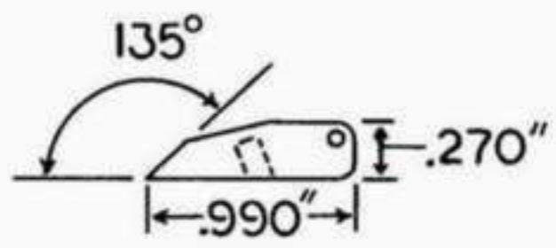
Fig. 3-24 TRIGGER LEVER
