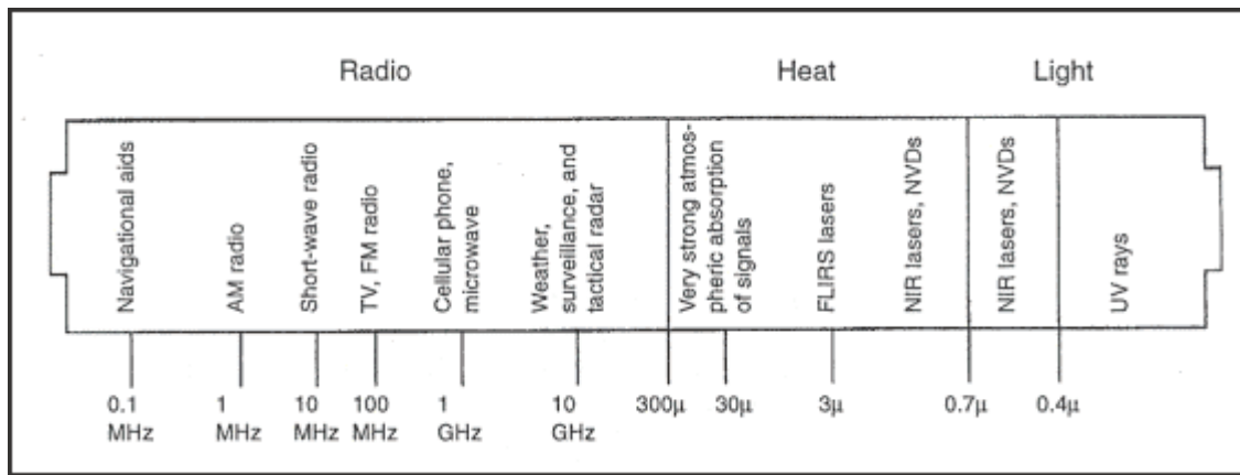
Figure 2-1. EM spectrum
