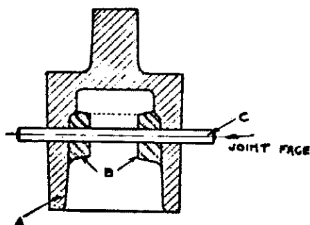
Fig. 10.—Piston
